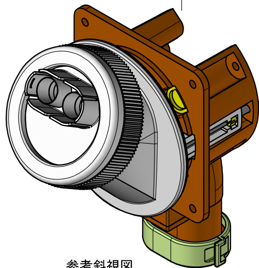
参考斜視図
